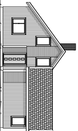
FASADE MOT NORDØST
