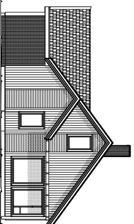
FASADE MOT SØRVEST
